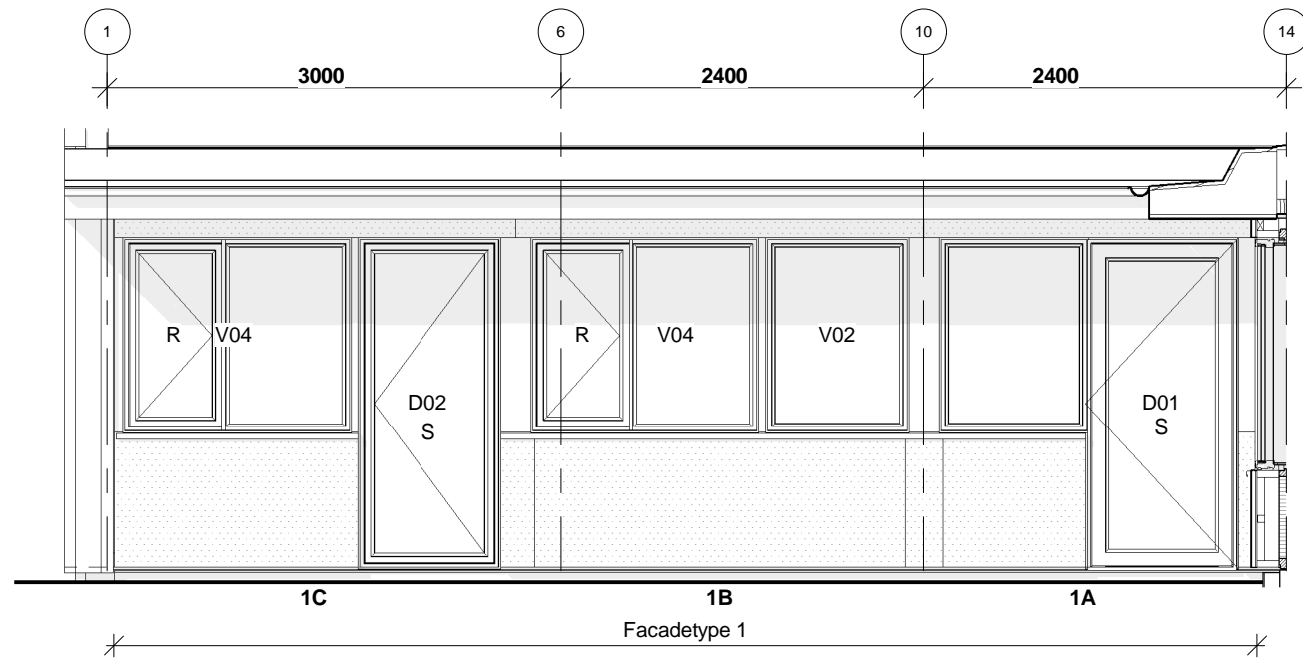
Let facade AN og BN, Syd
